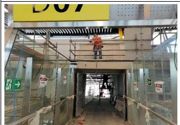
Espigón D: Estructuración cierre tabiques en accesos a puentes de embarque
