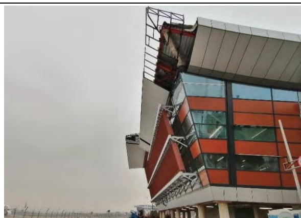
Espigón D: Instalación de soffito en cuerpo A
