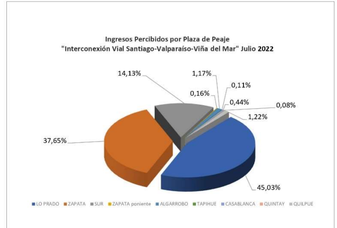
Gráfico 5: Ingresos Plaza de Peaje julio de 2022. Fuente: Datos Estadísticos proporcionados por SC y Validados por AIF.
