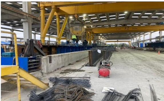
Ilustración N°5: Vigas Pretensada Puente Tijeral CD
