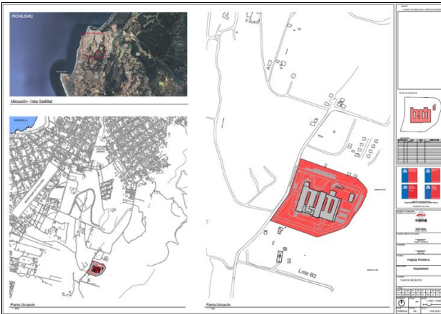
PLANTA DE UBICACIÓN HOSPITAL DE PICHILEMU
