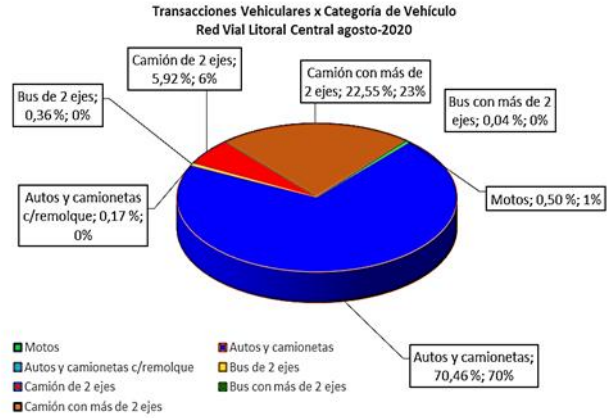
Gráfico 2: Flujos por Categoría de Vehículo, agosto 2020. Fuente: Estadística AIF.
