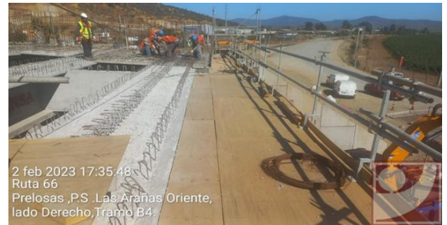
Paso Superior Las Arañas Oriente, Dm 92.542
