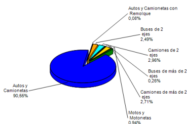
Gráfico 2: Distribución de Flujos por categoría de vehículo
