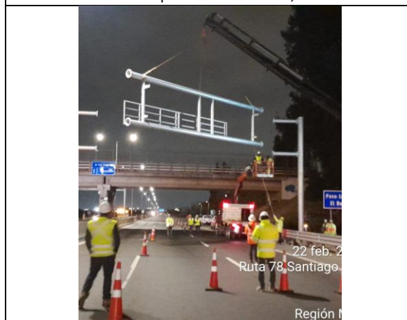
Instalación PMV- km.18,000- Desc
