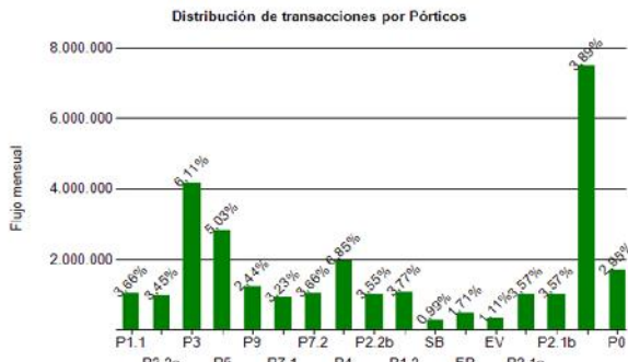
Gráfico 3: Distribución de Transacciones del Mes, por Pórtico de Cobro. Fuente: Informe 29 SICE, del 15.07.2022
