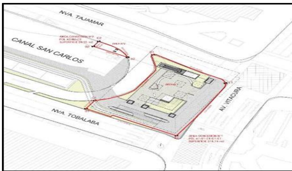
Planta emplazamiento Estación Sobre canal San Carlos
