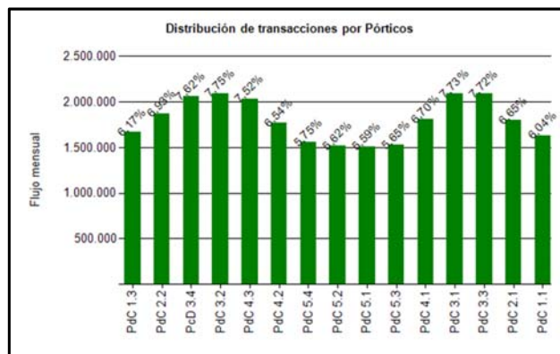
Gráfico 3: Distribución de Flujos por Pórtico de Cobro, noviembre 2018 Fuente: Reporte 29 SICE.
