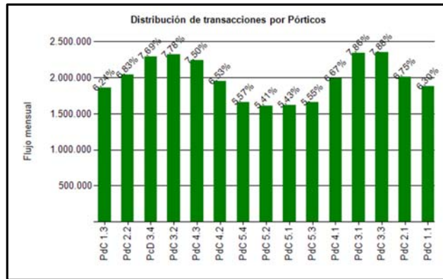
Gráfico 3: Distribución de Flujos por Pórtico de Cobro, diciembre 2019 Fuente: Reporte 29 SICE.
