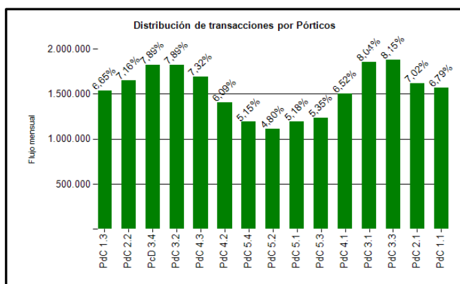
Gráfico 3: Distribución de Flujos por Pórtico de Cobro, febrero 2024. Fuente: Reporte 29 SICE.
