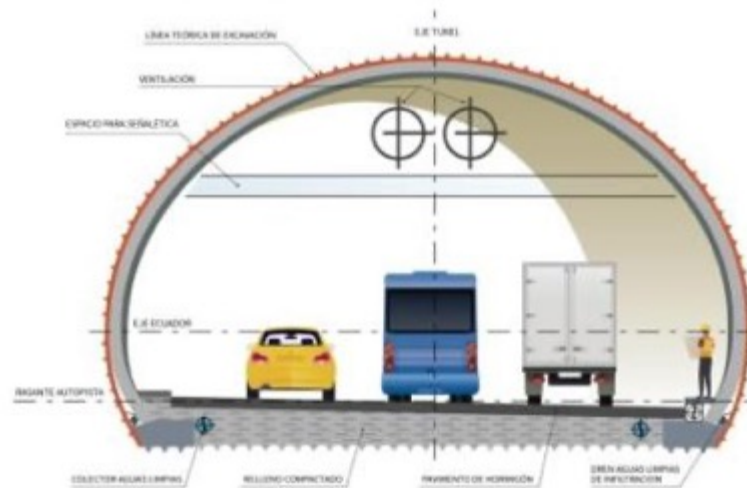
Esquema diseño de túneles Ruta 68. Información en desarrollo en estudio integral
