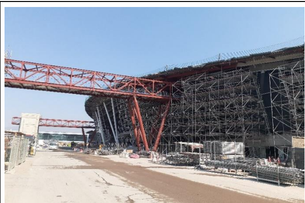
Vista fachada sur del T2M y Pasarelas
