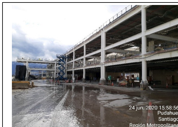
T1A: Calle de servicio lado Sur, vista lado Oriente a Poniente.
