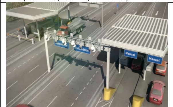
Maqueta Virtual, Ruta F-20, Pórtico telepeaje Free Flow y Caseta de Cobro Manual, Dm 6.500
