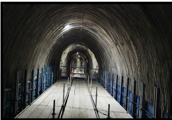
FIG N°5: Vista General Túnel de Desvío - Portal Salida
