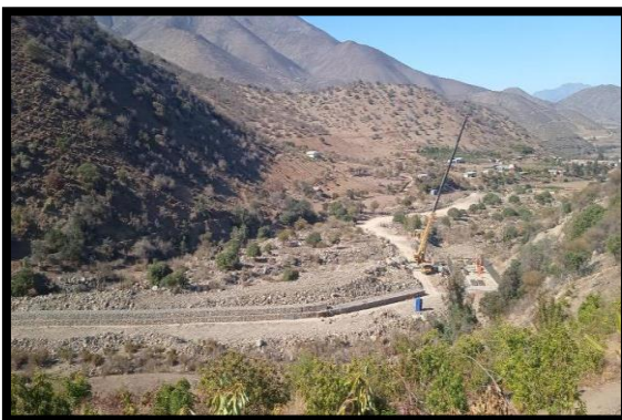
FIG N°11: Estación Fluviométrica Las Carditas – Construcción Muro de Contención
