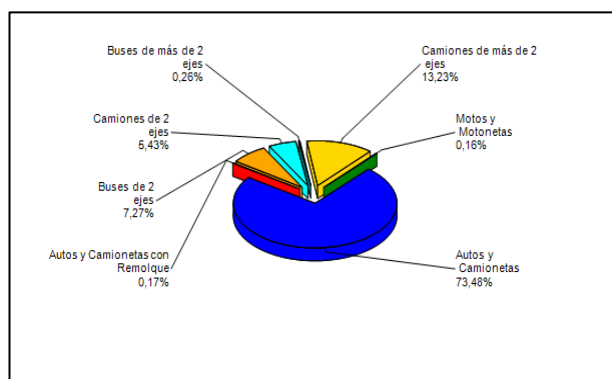
Gráfico 2: Distribución de Flujos por categoría de vehículo Fuente: Reportes SICE Agosto 2016
