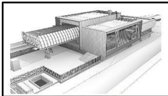
Estación Santa Clara – nuevo Layout (En Ciudad Empresarial – Huechuraba- Incluye almacén de cabinas)
