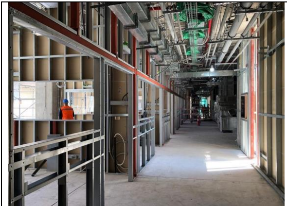
Estructura de acero galvanizado tabiques y pilares P2 entre ejes 21-22/M-P; 27-28/K-L HDS
