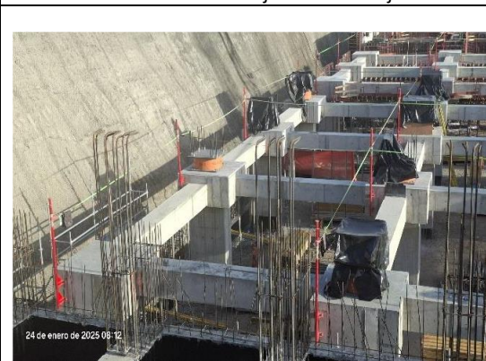
Rellenos de mejoramiento Bajo Radier
