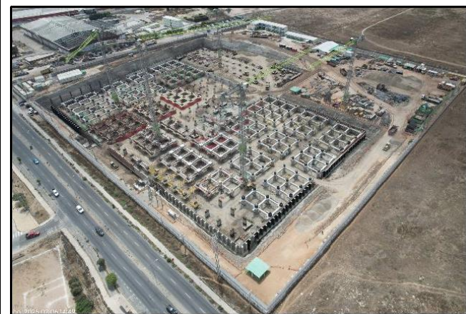
Instalación de Aisladores sísmicos
