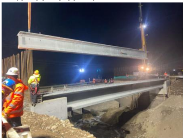
Montaje vigas y armado Losa Puente ELC-1 en B2
