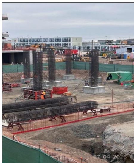
Fundaciones edificio industrial
