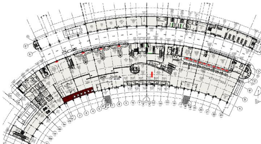
Layout: "Servicio de Información: Monitores FIDS - Primer Piso"
