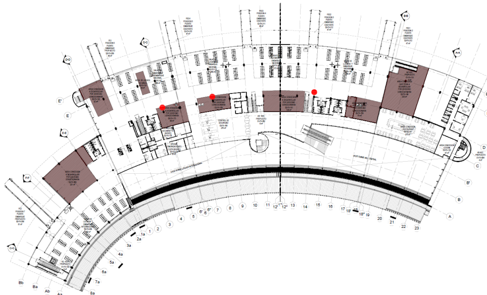
Layout: "Servicio de Conexión Inalámbrica a Internet segundo nivel"
