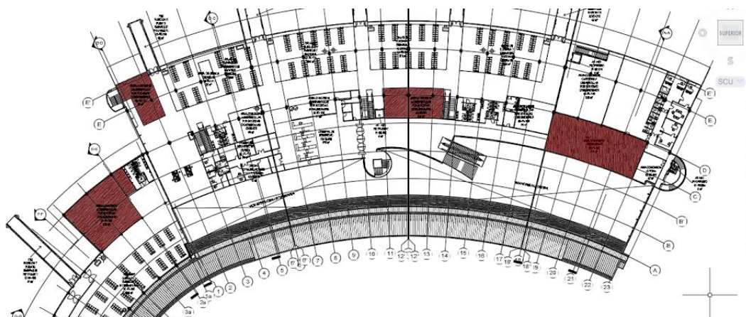
Layout: “Servicio de Alimentación y Bebida – Segundo Piso”
