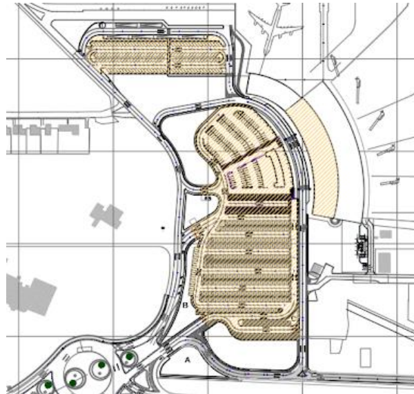
Layout: "Servicio de Vigilancia – Áreas Públicas"
