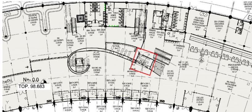
Layout: "Centro de Atención al Público"
