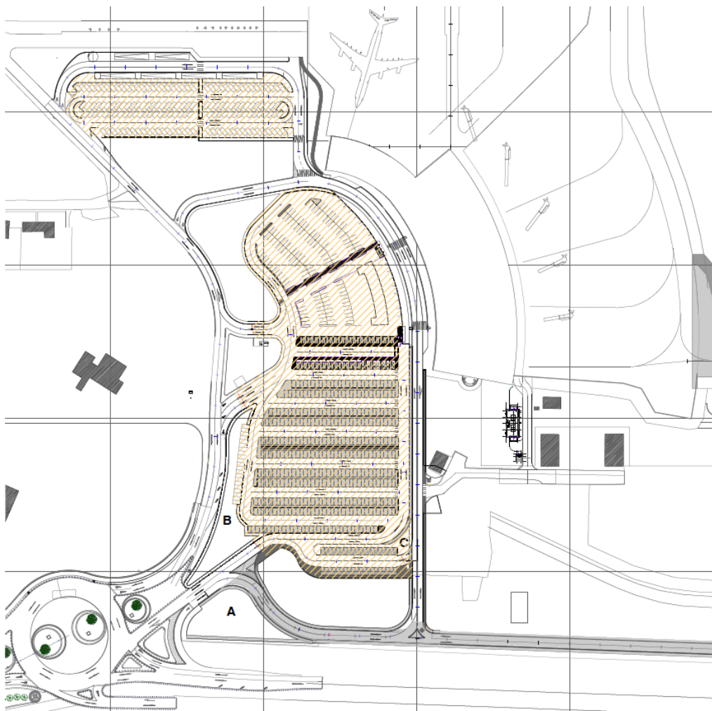
Layout: "Estacionamientos Públicos para Vehículos en General"
