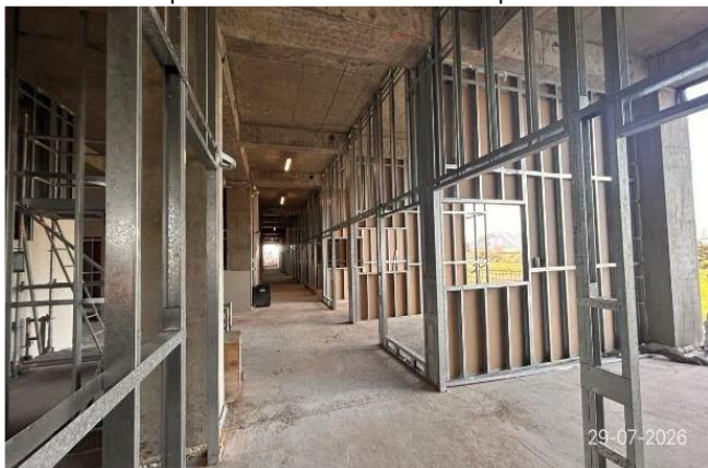
Avance de tabiquerías interiores Edificio Principal
